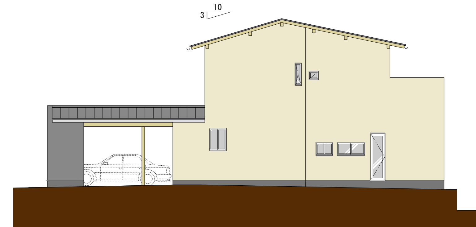
西立面図
