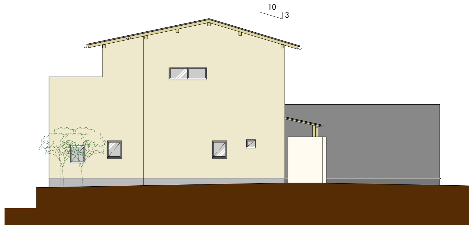
東立面図
