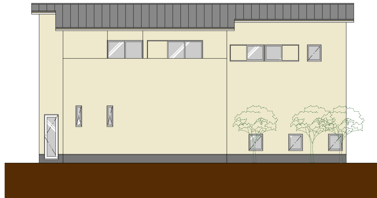
南立面図
